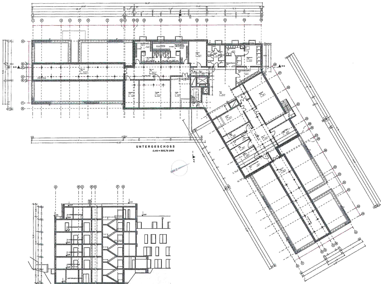
SCHNITT A-A
