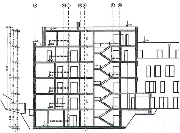
SCHNITT A-A
